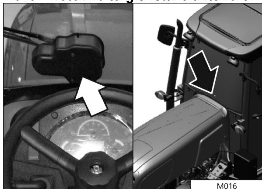
M016 - Motorino tergilavaggio anteriore
