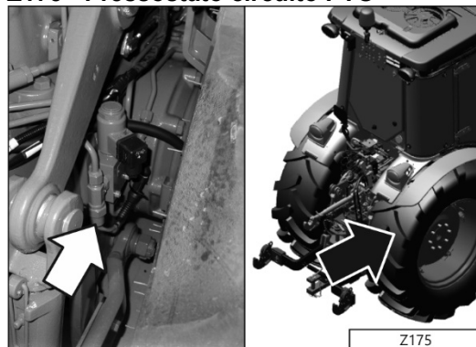
Z175 - Pressostato circuito PTO
