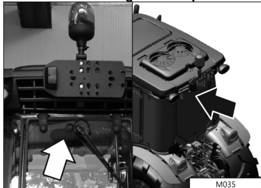
M035 - Motorino tergilavaggio posteriore
