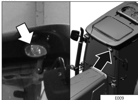
E009 - Luce di lavoro anteriore sinistra su tetto
