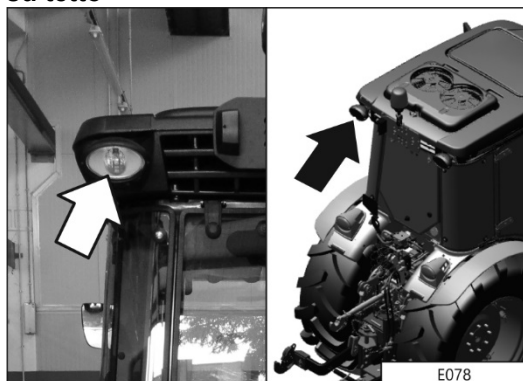
E078 - Luce di lavoro posteriore sinistra su tetto
