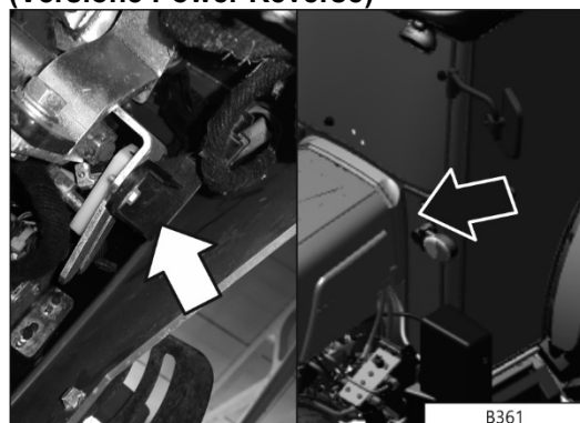
B385 - Sensore pressione marcia bassa (Versione Power Reverse)
