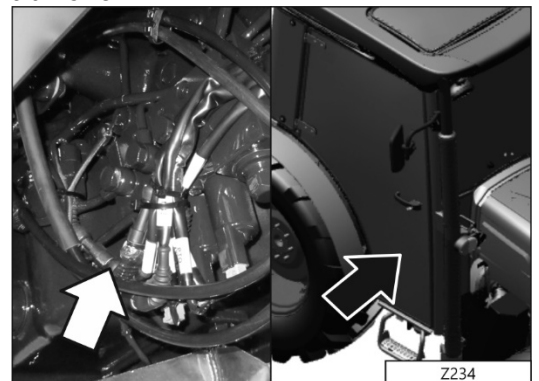
Z234 - Pressostato circuito doppia trazione
