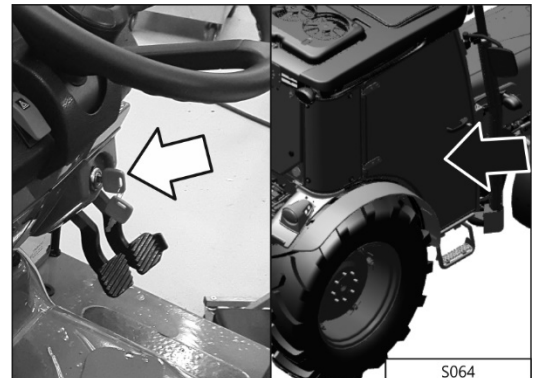
S064 - Interruttore di accensione
