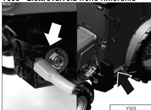
Y503 - Elettrovalvola freno rimorchio
